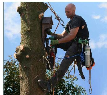
DRUCKLUFT MOBILO
