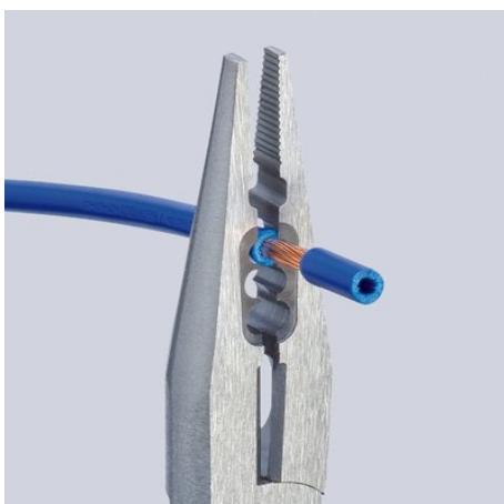
Abisolieren 0,5 - 0,75 / 1,5 / 2,5 m 2
