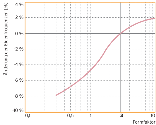
Abb. 8: Eigenfrequenzen*
