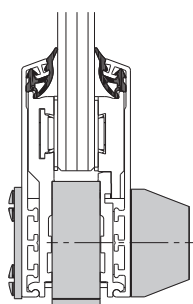
Halbzylinder
