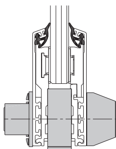
Doppelzylinder
