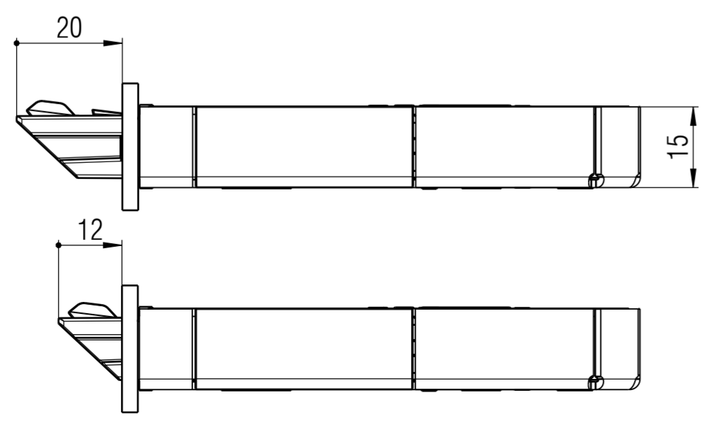
Fallenriegel verriegelt
